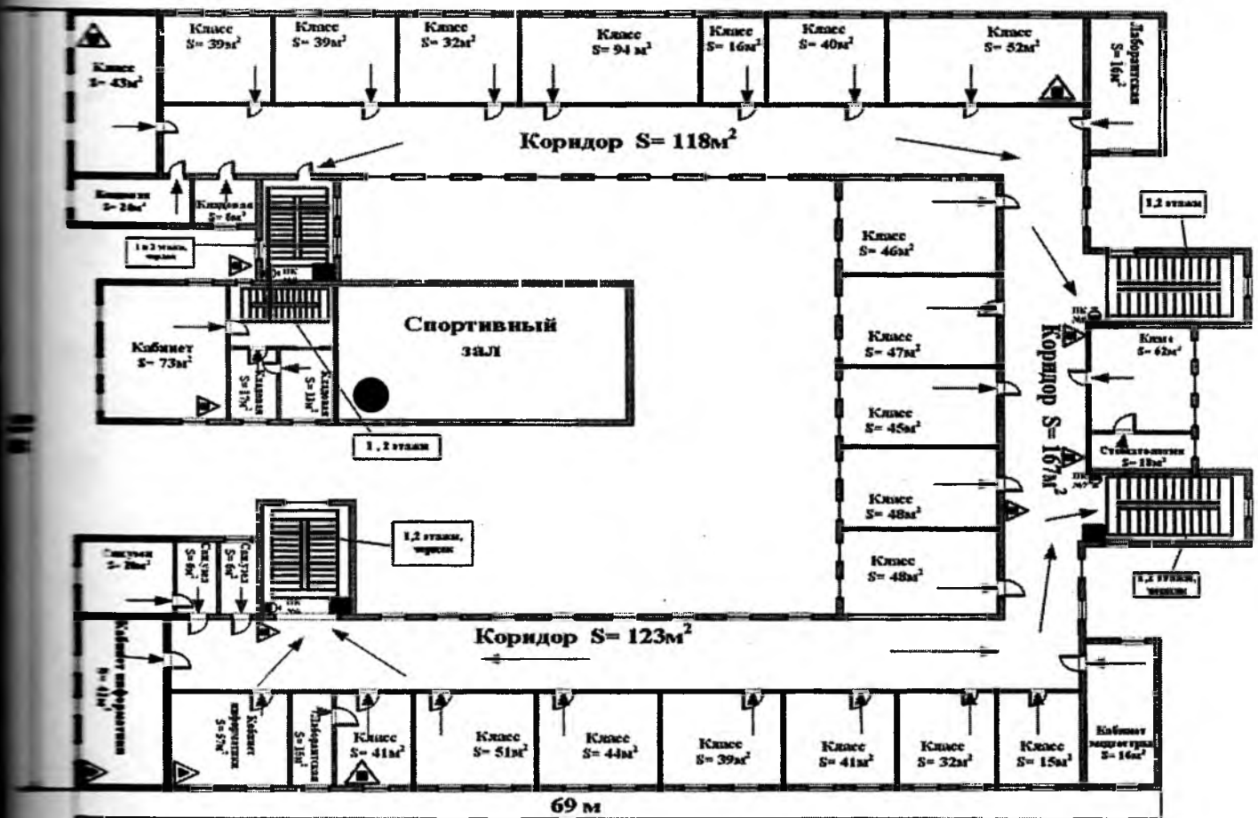
Рис. 2-го этажа здания
